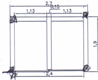
VISTA EN PLANTA DIMENSIONADA
