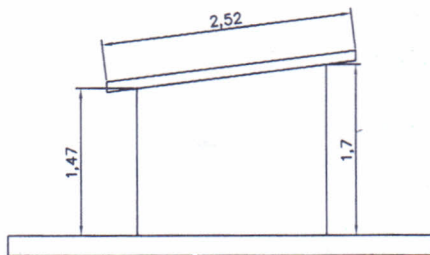
ELEVACION LATERAL DIMENSIONADA
